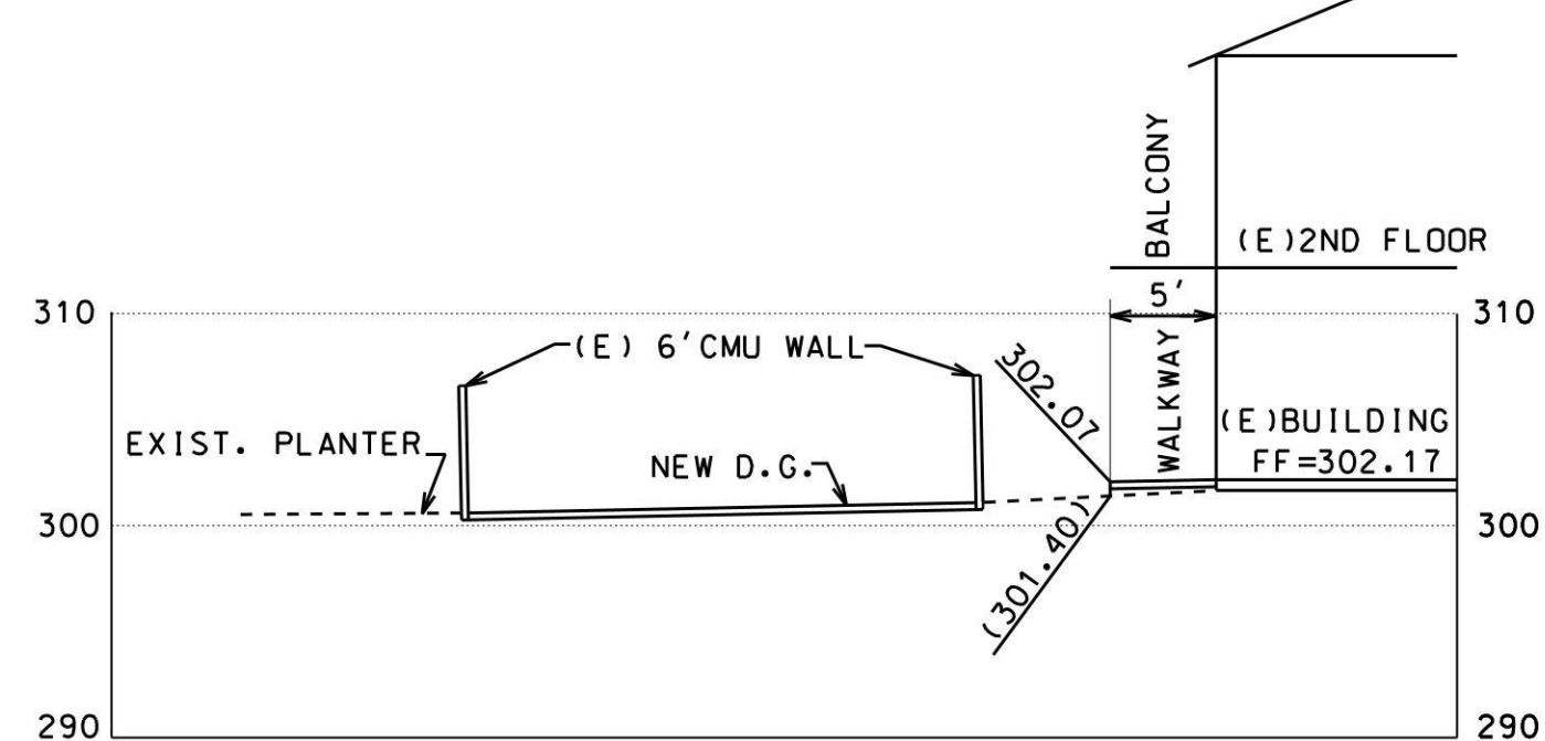
SECTION D-D
